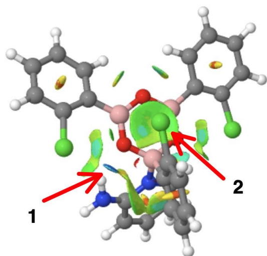
2-aminopyridine
